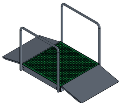
Grep 1a
