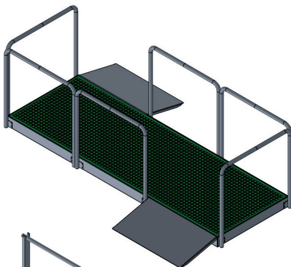
Grep 3
