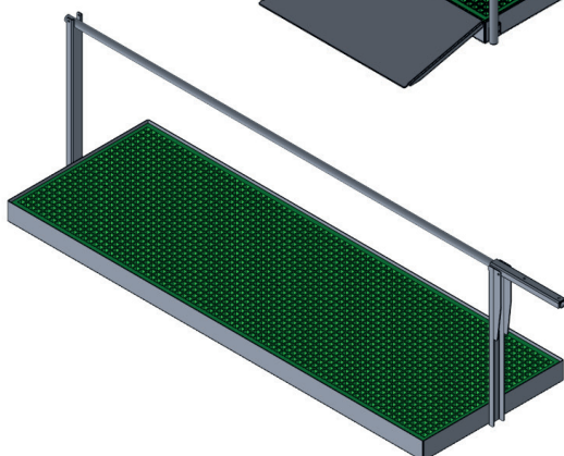
Grep 4
