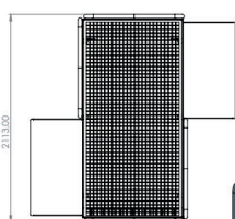
Grep 2
